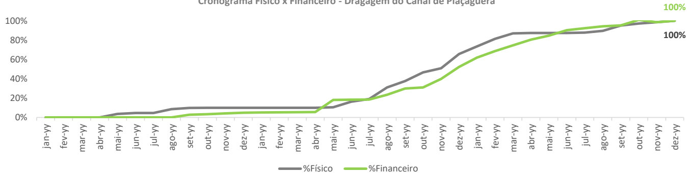
Cronograma Físico x Financeiro - Dragagem do Canal de Piaçaguera
