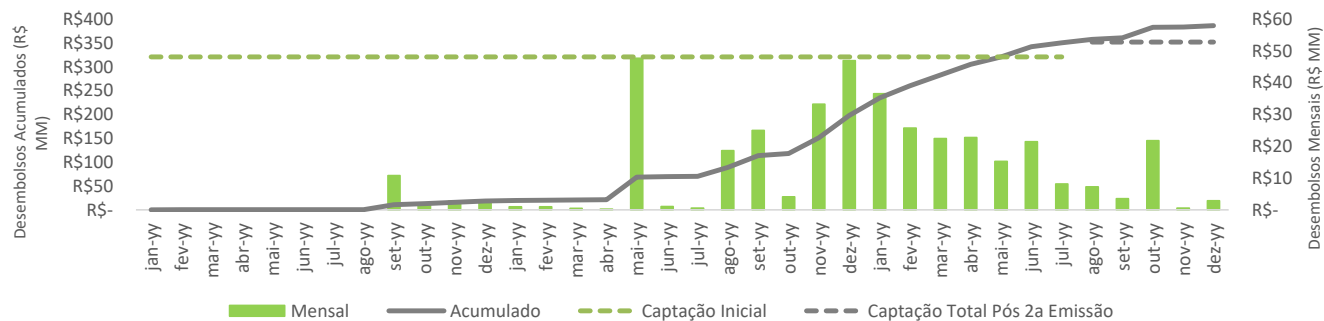
Cronograma Financeiro - Projeto Dragagem do Canal de Piaçaguera
